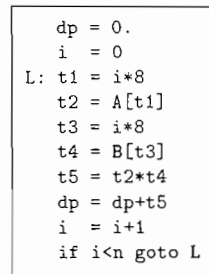
图 9-11 计算点积的中间代码
