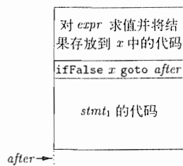
图 2-42 if 语句的代码布局
