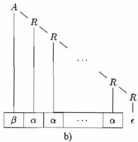
图 2-20 生成一个串的左递归方式和右递归方式
