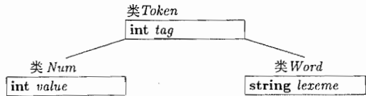
图 2-32 类 Token 以及子类 Num 和 Work
