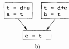
图 9-6 在公共子表达式消除过程中引入的复制语句
