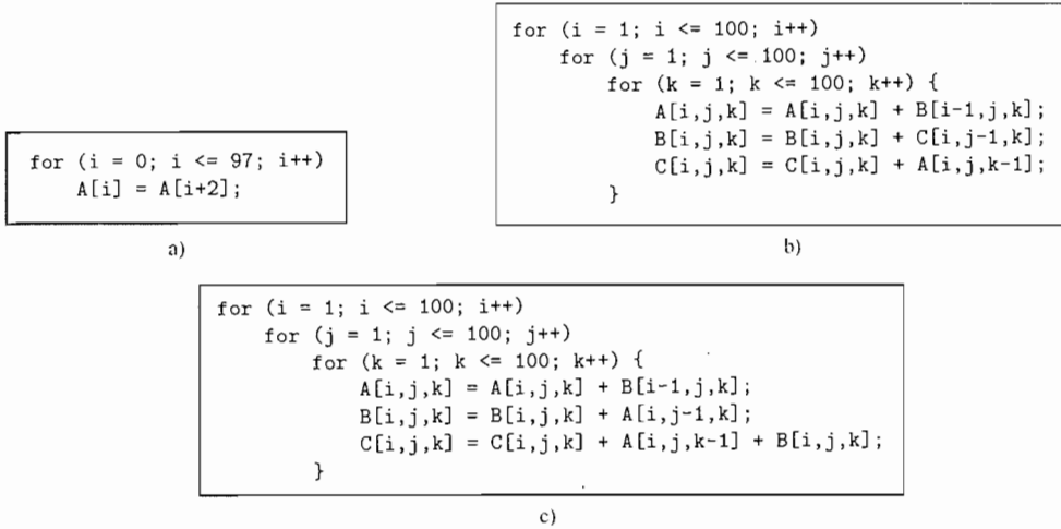
图 11-37 练习 11.7.2 的代码
