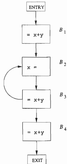
图 9-37 练习 9.5.1 的流图
