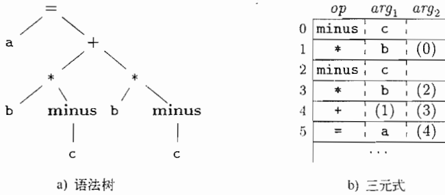
图 6-11 a = b * -c + b * -c 的表示
