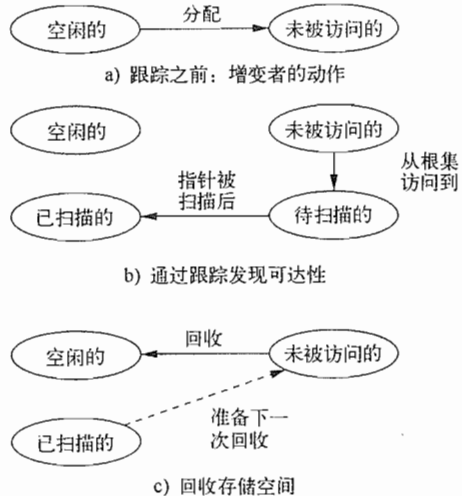
图 7-23 在一个垃圾回收循环中的存储块的状态
