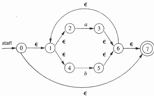
图 3-45 r_5 的 NFA
