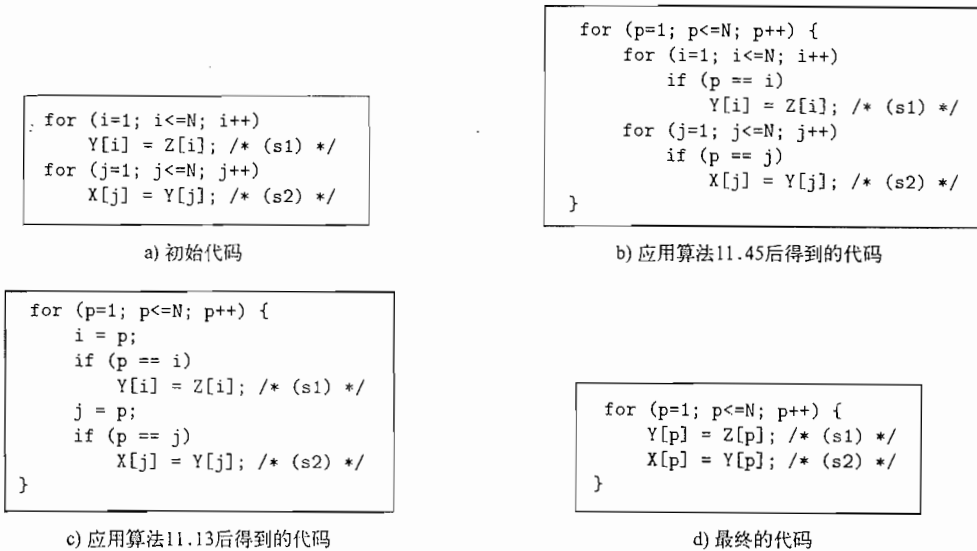
图 11-30 例 11.46 的代码
