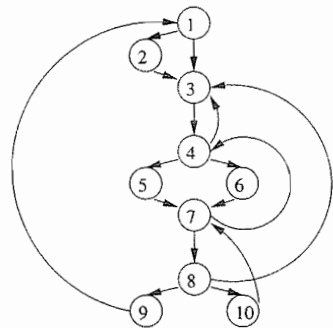
图 9-38 一个流图
