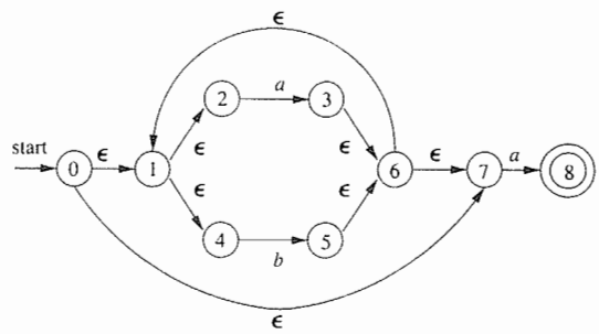
图 3-46 r_7 的 NFA
