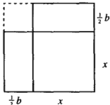
图 5-1 配方
