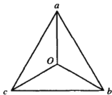
图 3-3 仿射平面
