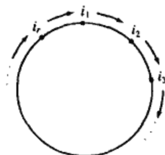
图 2-8 一个循环
