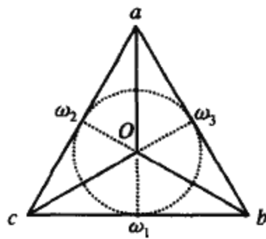
图 3-4 射影平面
