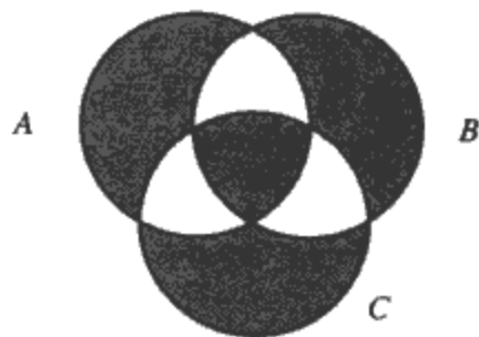
图 2-7 结合律
