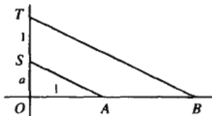
图 4-4 a^{-1}
