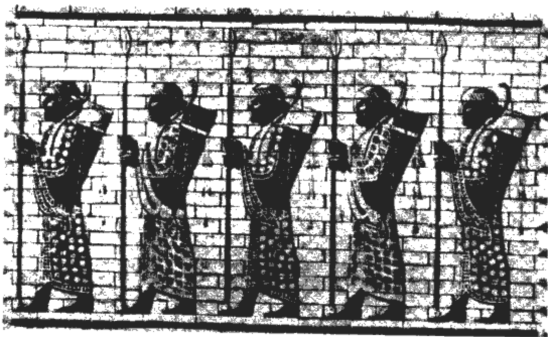
图 6-4 波斯弓箭手
