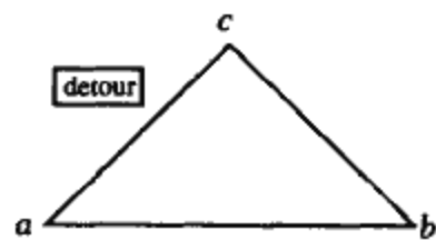
图 4-8 三角不等式
