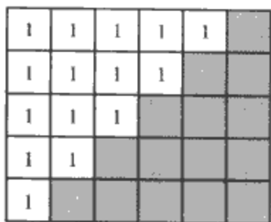
图 1-2 1+2+\cdots+n = \frac{1}{2}n(n+1)
