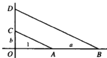
图 4-3 ab
