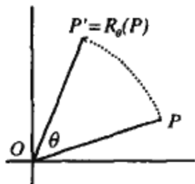
图 2-11 旋转
