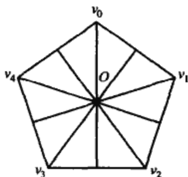
图 2-15 \pi_5 的对称
