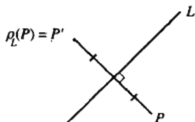
图 2-12 反射
