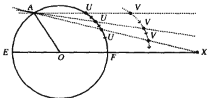
图 4-6 米尺滑动
