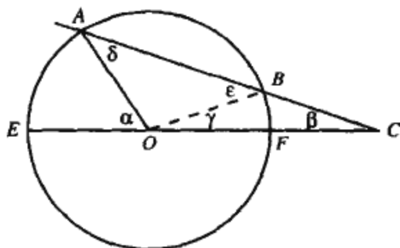
图 4-7 三等分 \alpha
