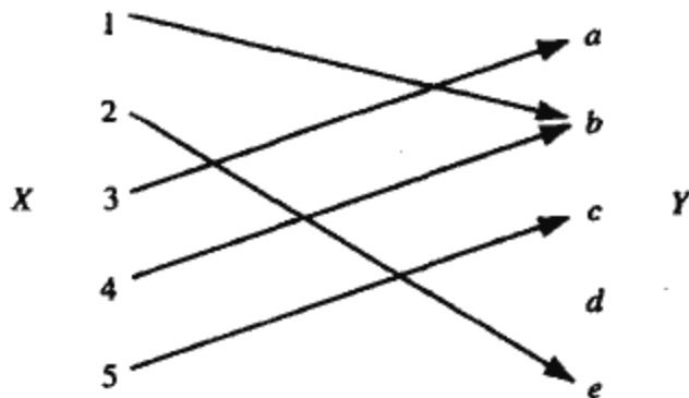
图 2-4 一个函数
